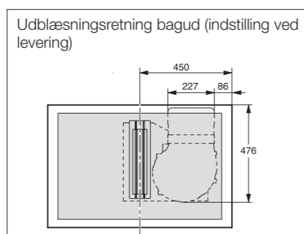
KMDA 7634 FL – Uden stålramme, planforsænket i 600 mm dyb bordplade
