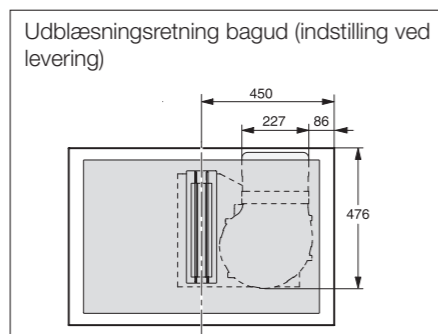
KMDA 7634 FR – Med stålramme, monteret oven på 600 mm dyb bordplade
