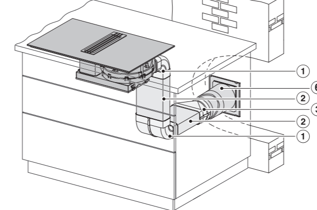
Eksempel D >600 mm dyb bordplade.
