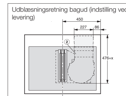
KMDA 7634 FL – Uden stålramme, monteret oven på >600 mm dyb bordplade
