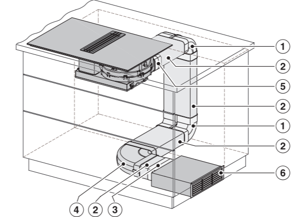
Eksempel F >600 mm dyb bordplade.
