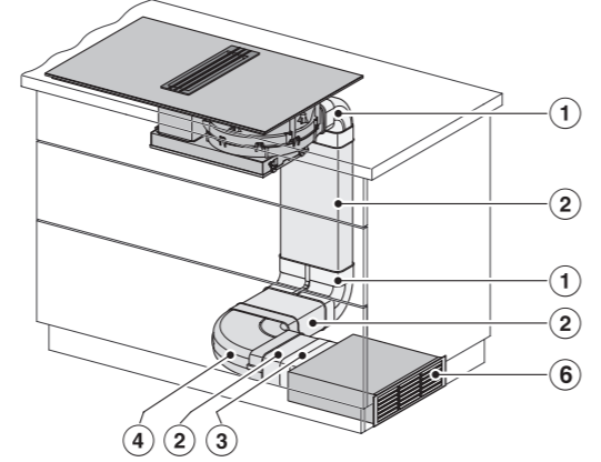
Eksempel A 600 mm dyb bordplade.
