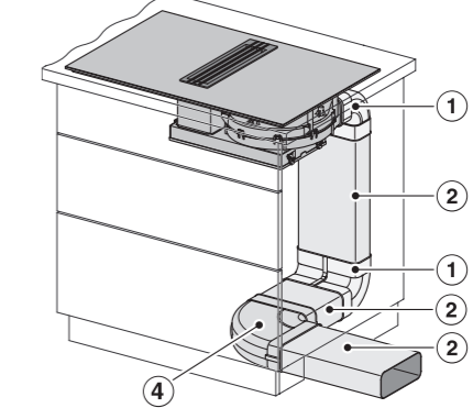
Eksempel G 600 mm dyb bordplade.
