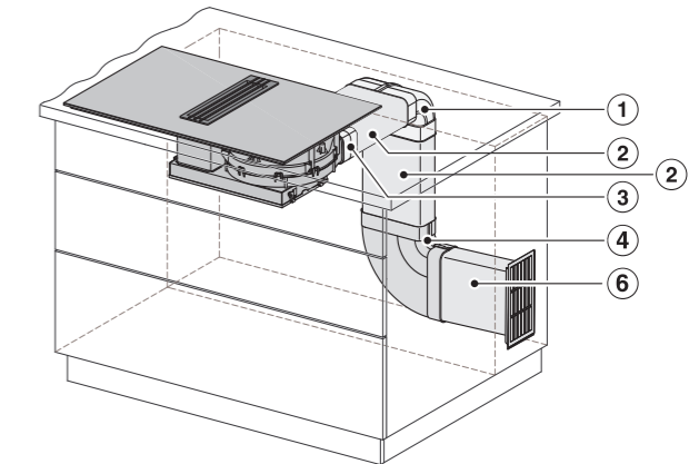
Eksempel I >600 mm dyb bordplade.
