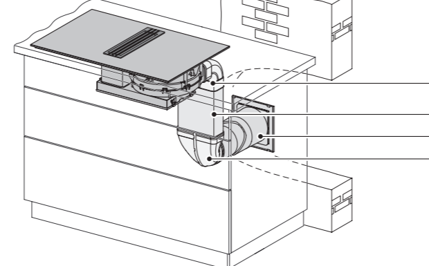
Eksempel C 600 mm dyb bordplade.
