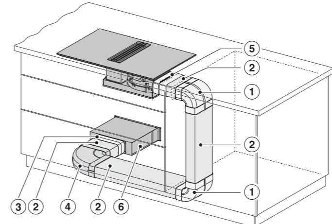
Eksempel E >600 mm dyb bordplade.
