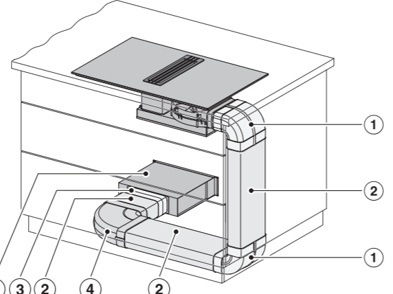
Eksempel C >600 mm dyb bordplade.
