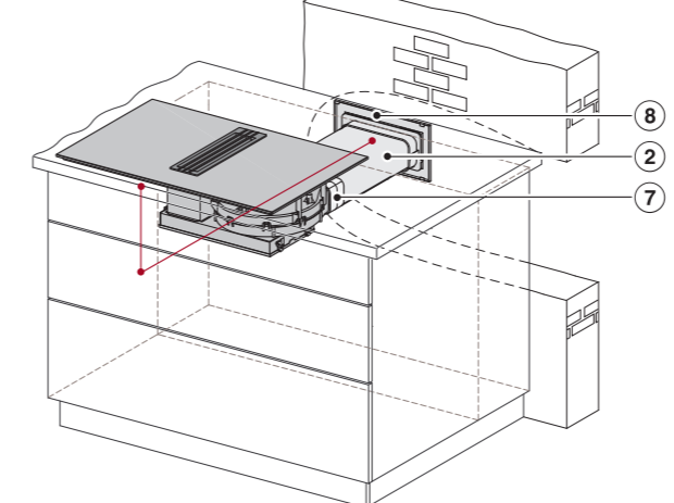
Eksempel E >600 mm dyb bordplade.
